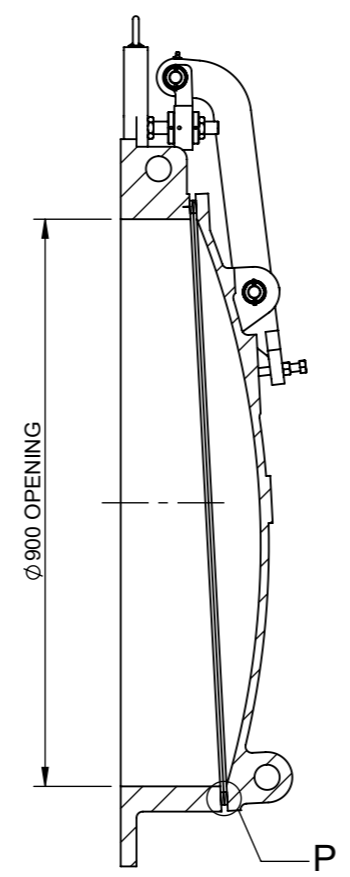
SECTION A-A
