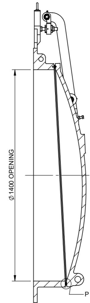
SECTION A-A
